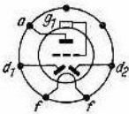
СБ-156
